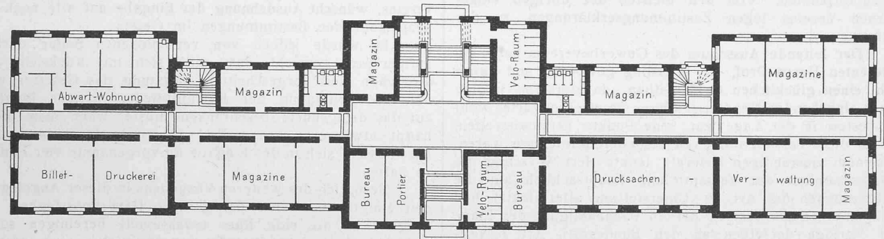
Grundriss vom Erdgeschoss. — Masstab 1 : 500.
