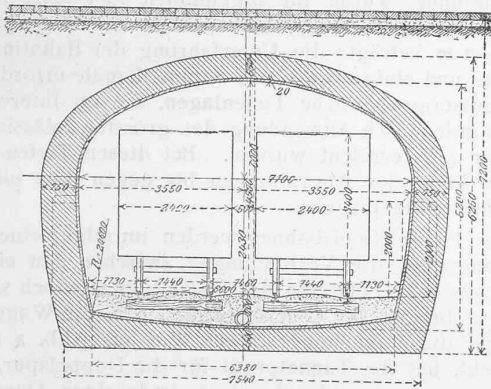
Abb. 2. Normalprofil des zweisepurigen Tunnels. Masstab 1 : 150.
