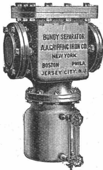
Oel- und Wasser- Abscheider.
