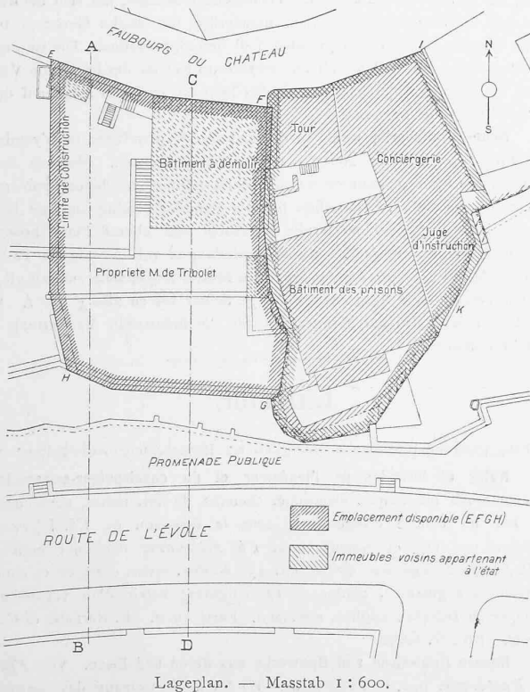
Lageplan. — Masstab 1 : 600.
