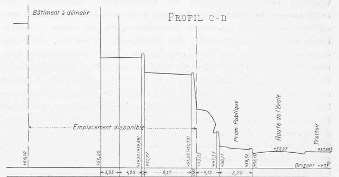
Querprofile. — Masstab 1 : 600.
