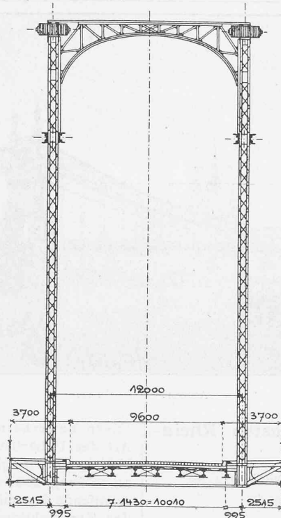
1 : 300. Abb. 4. Schnitt bei 15 u. 18.
