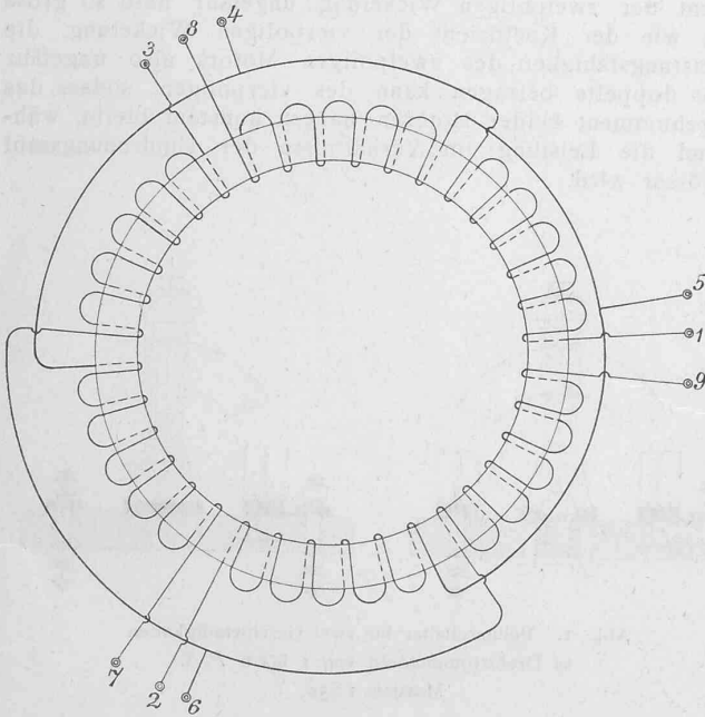
Abb. 3. Wickelungs- und Schaltungsdiagramm für Drehstrommotoren mit zwei Geschwindigkeiten. Zwei- und vierpolig.
