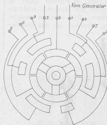
Abb. 3. Wickelungs- und Schaltungsdiagramm für Drehstrommotoren mit zwei Geschwindigkeiten. Zwei- und vierpolig.
