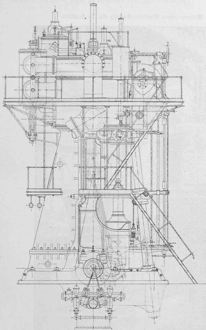
Abb. 4. Seitenansicht. — Masstab 1:75.
