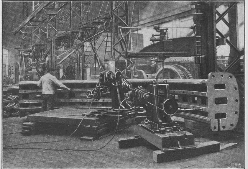
Abb. 14. Bohren eines Gehäuseviertels mit zwei tragbaren Bohrmaschinen.
