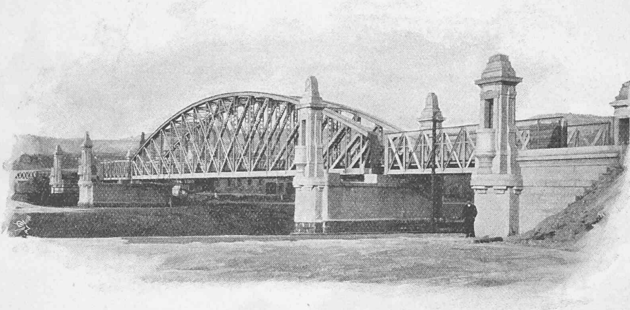
Abb. 16. Donaukanalbrücke. — Heiligenstadt-Brigittenau.
