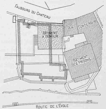
Lageplan. — Masstab 1 : 1000.
