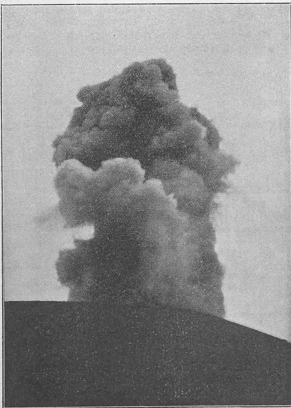
Abb. 24. Eruptionswolke des Vesuvs. Nach einer Aufnahme des Herrn Mateucci, Direktor des Observatoriums, vom 19. März 1903.
