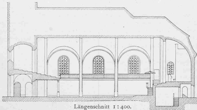
Längenschnitt 1 : 400.
