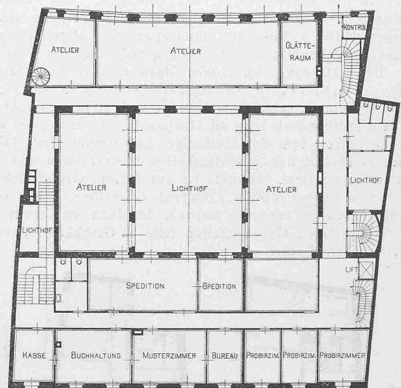
Abb. 16. Grundriss vom zweiten Stock. — 1:400.
