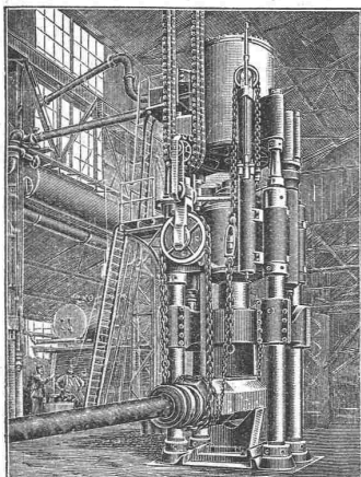
Dampfhdraulische Schmiedepresse.
