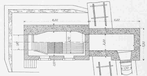
Abb. 13. Grundriss, Quer- und Längsschnitt vom Wasserschloss. Masstab 1:250.
