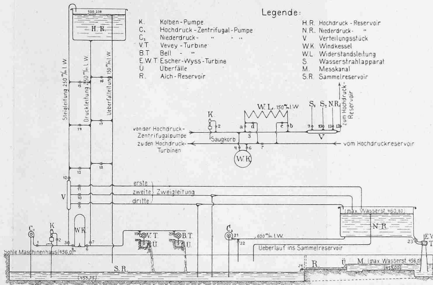
Abb. 25. Schema der Anordnung der hydraulischen Abteilung.
