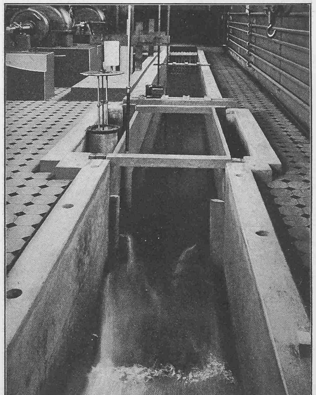
Abb. 23. Ansicht des Messkanals gegen die Durchflussrichtung.
