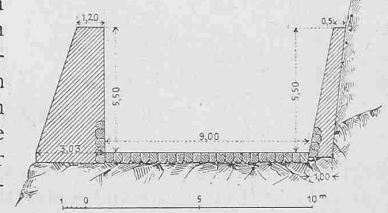
Abb. 7. Querprofil des Ueberlaufkanals. — 1:300.
