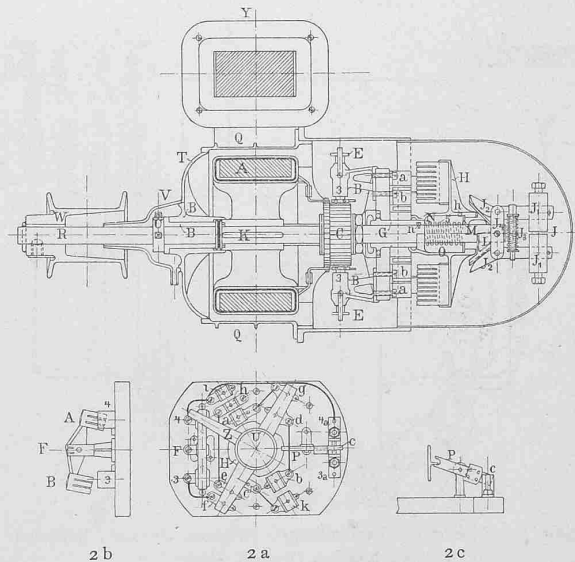
Abb. 2. Dynamo mit automatischem Regulator. — System Stone.
