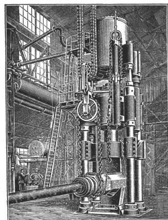
Dampfhydraulische Schmiedepresse.
