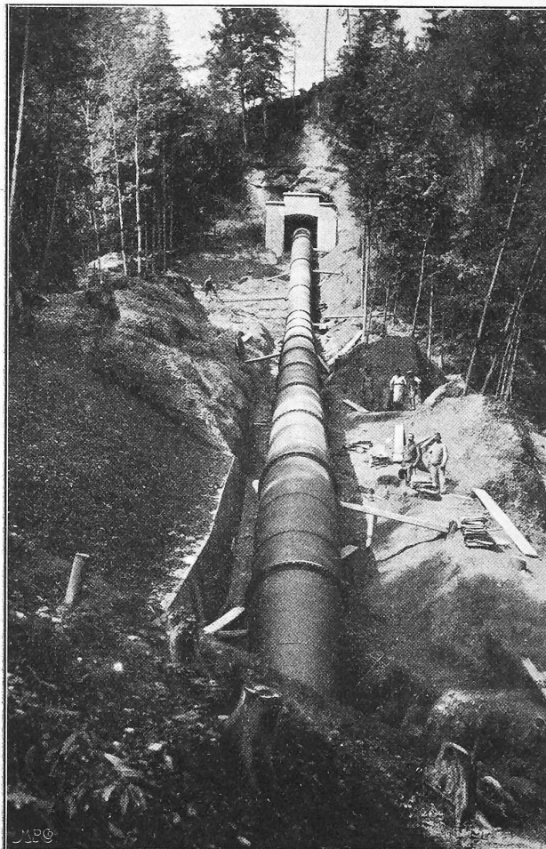
Abb. 30. Mittlerer Teil der Druckleitung.
