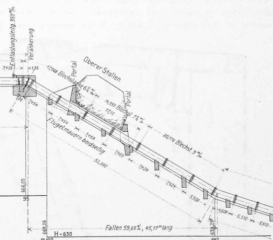
Abb. 28a. Längenprofil des oberen Teils der Druckleitung. — Masstab 1:800.
