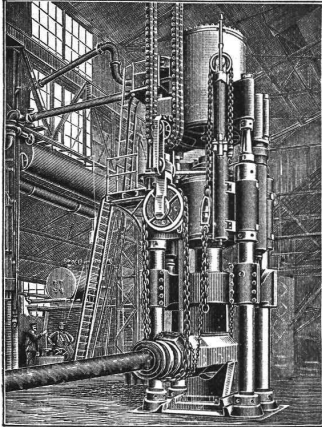
Dampfhdraulische Schmiedepresse.
