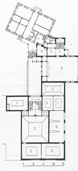
Grundriss vom Obergeschoss. I: 1000.
