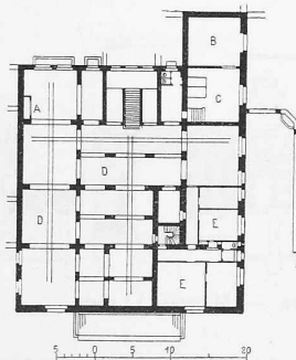
Grundriss vom Untergeschoss. I: 1000.
