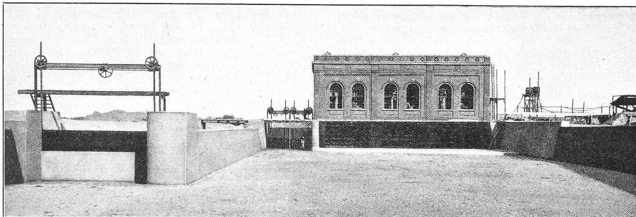
Abb. 4. Turbinenanlage der Spinnerei am Stadtbach in Augsburg. — Ansicht des Turbinenhauses und der Fallen vom Zulaufkanal aus.
