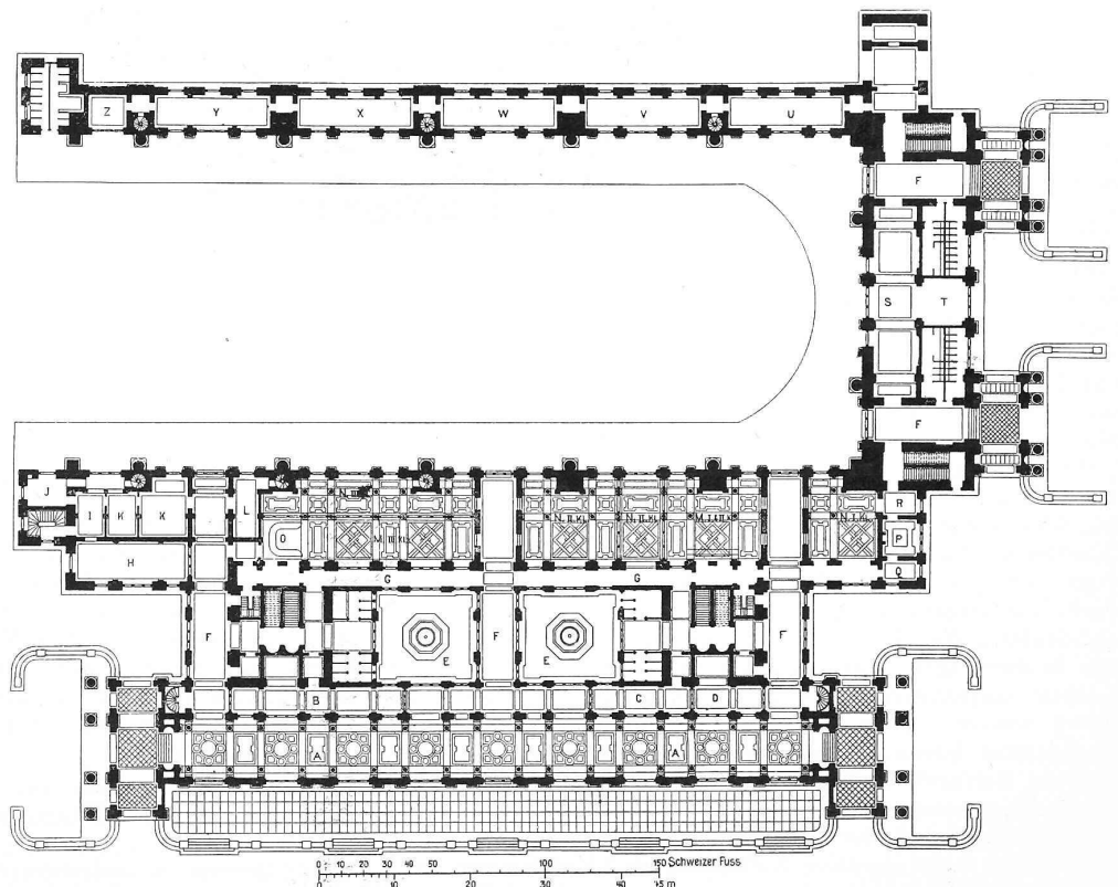
Abb. 2. Grundrissentwurf für das Bahnhofgebäude in Zürich. — Masstab 1 : 1000.
