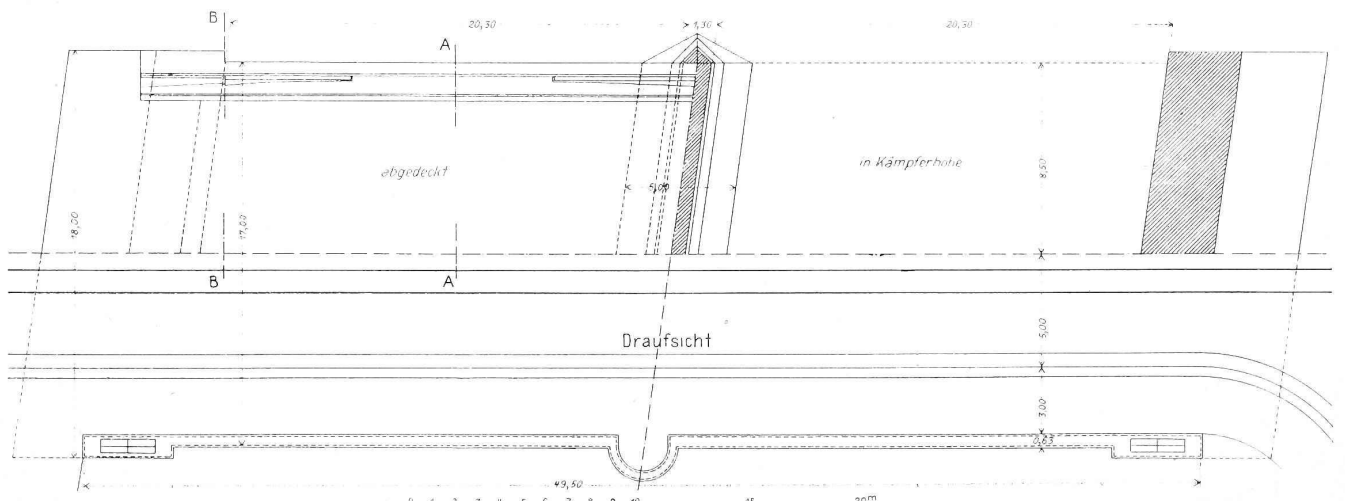
Längsschnitt und Grundriss. — Masstab 1 : 300.
