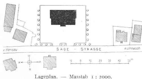
Lageplan. — Masstab 1 : 2000.
