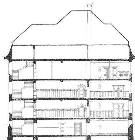
Längsschnitt. — Masstab 1 : 400.
