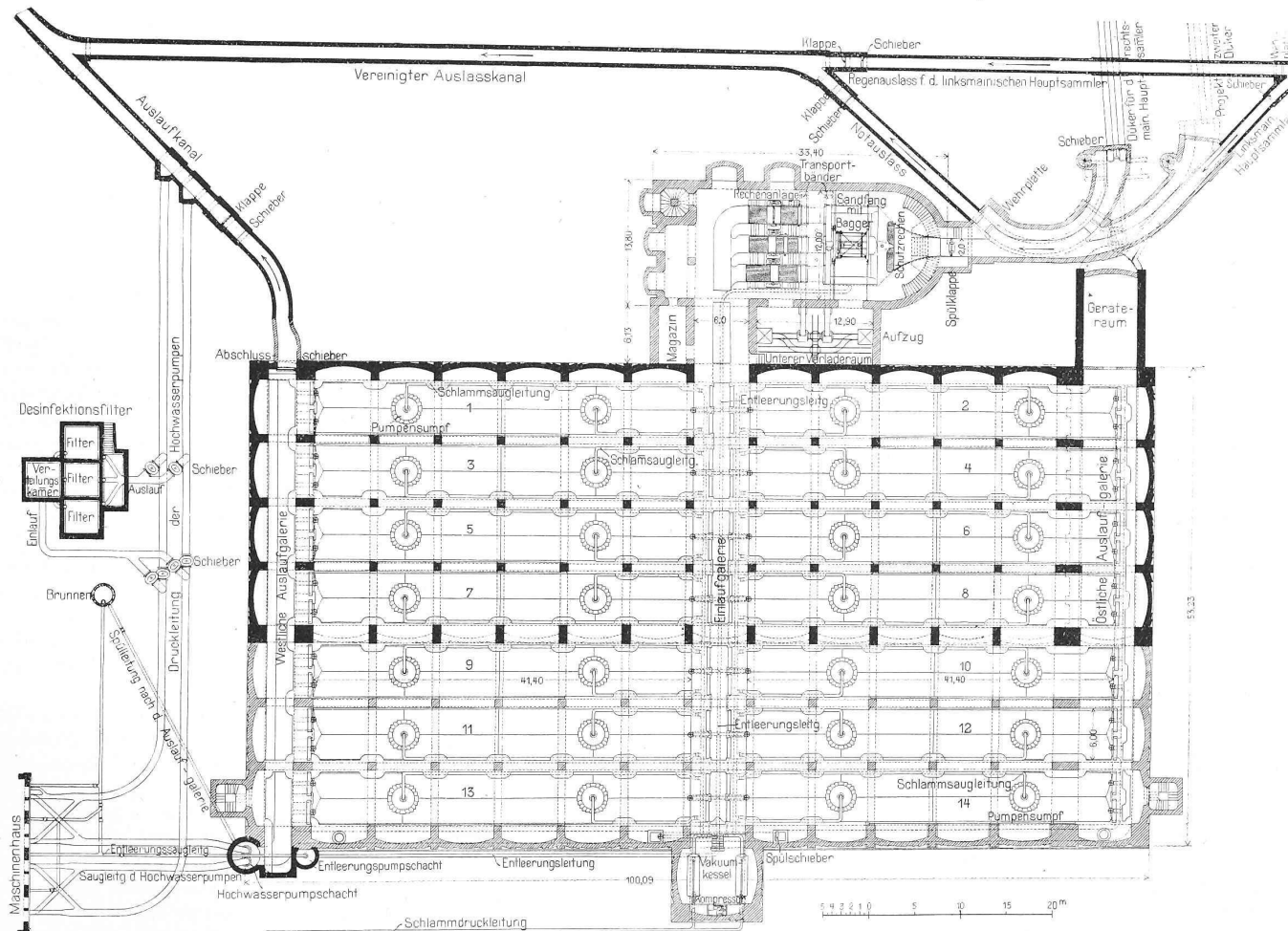
Abb. 2. Grundriss der Kläranlage nach dem Umbau und der Erweiterung. — Masstab 1:700.
