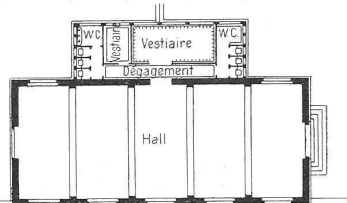
Ansicht und Grundriss der Turnhalle. — 1:600.
