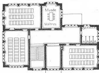
Grundriss vom I. Obergeschoss. — 1:600.
