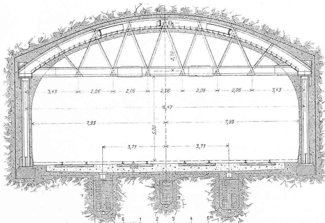
Abb. 26. Profil der viergeleisigen Strecke des Tunnels unter dem North River. — Masstab 1 : 200.
