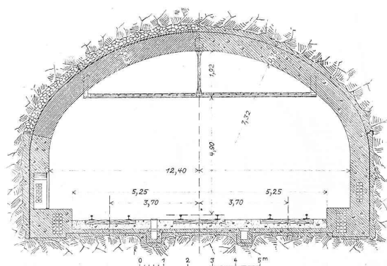
Abb. 27. Normalprofil des dreigeleisigen Tunnels in Manhattan. Masstab 1 : 200.
