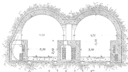
Abb. 28. Normalprofil des Zwillingstunnels in Manhattan. Masstab 1 : 200.
