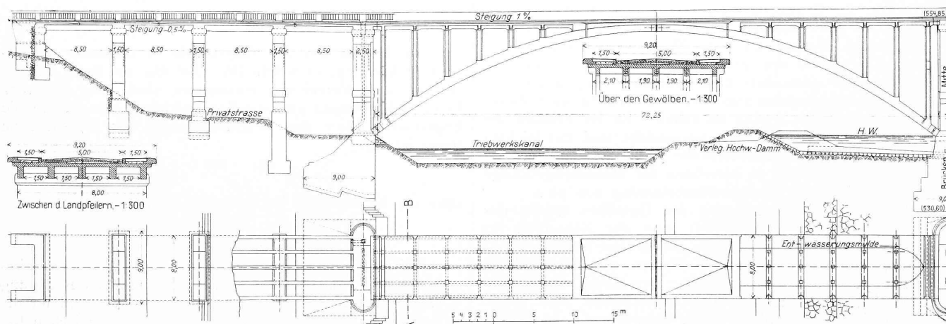
Abb. 4. Längsschnitt und Grundriss der Isarbrücke bei Grünwald. Linke Hälfte. — Masstab 1:600.
