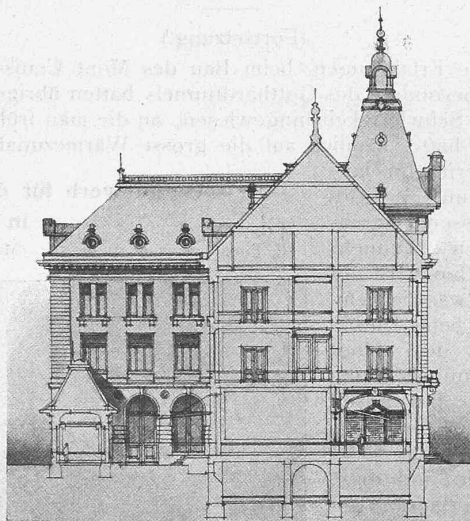
Querschnitt durch den Mittelbau. — 1:600.
