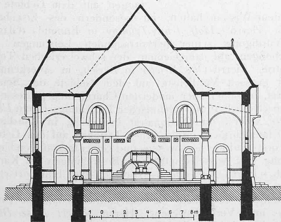
Querschnitt durch die Kirche. — Massstab 1 : 300.
