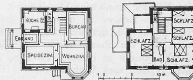
Grundrisse vom Erdgeschoss und Obergeschoss des Pfarrhauses. — Massstab 1 : 600.
