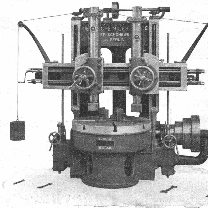
Karussell-Drehbank von 1000 mm Durchmesser.
