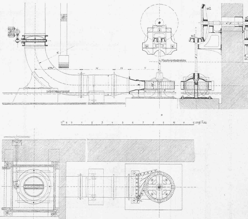
Abb. 1. Tangentialrad für Laiblin & Elben in Pfullingen. — 1:60. Gebaut von Escher Wyss & Cie. 1847.
