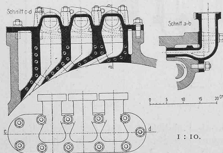
Abb. 2. Düsenapparat.
