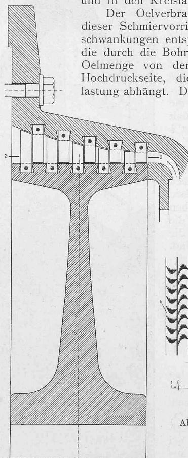
Schaufelung im Schnitt a-b.
