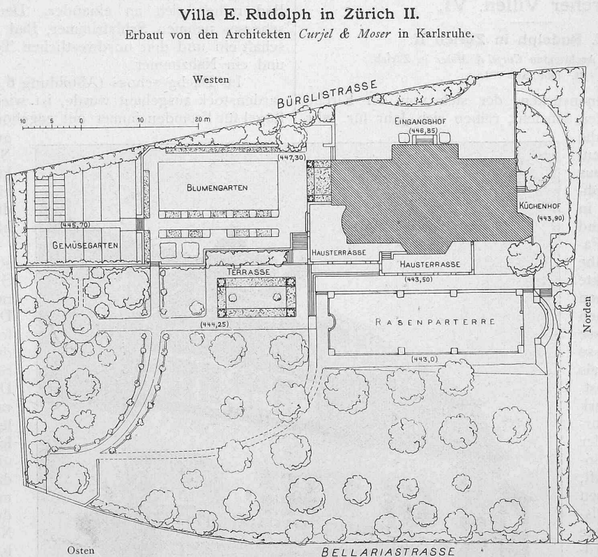
Abb. 2. Lageplan. — Masstab 1:800.
