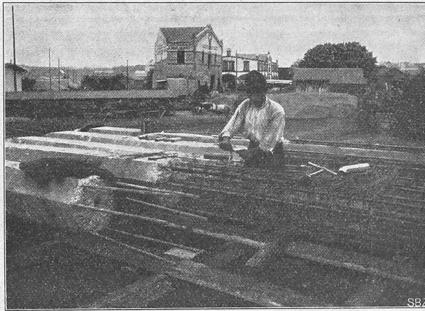
Abb. 24. Aufstücken von Hennebique-Pfählen.
