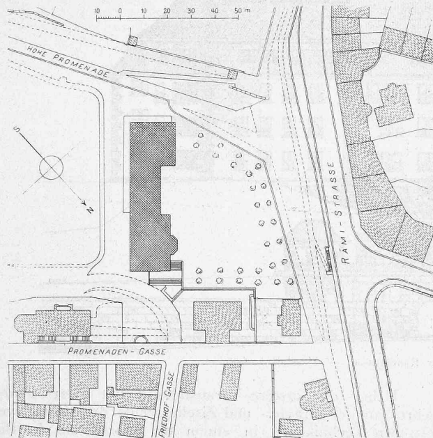
Lageplan. — Masstab 1 : 2000.
