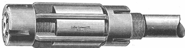
Nachstellbare Reibahle.
