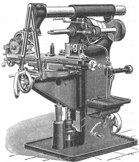
Universal-Fräsmaschine. No. 2.
