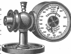
Handtachometer.
