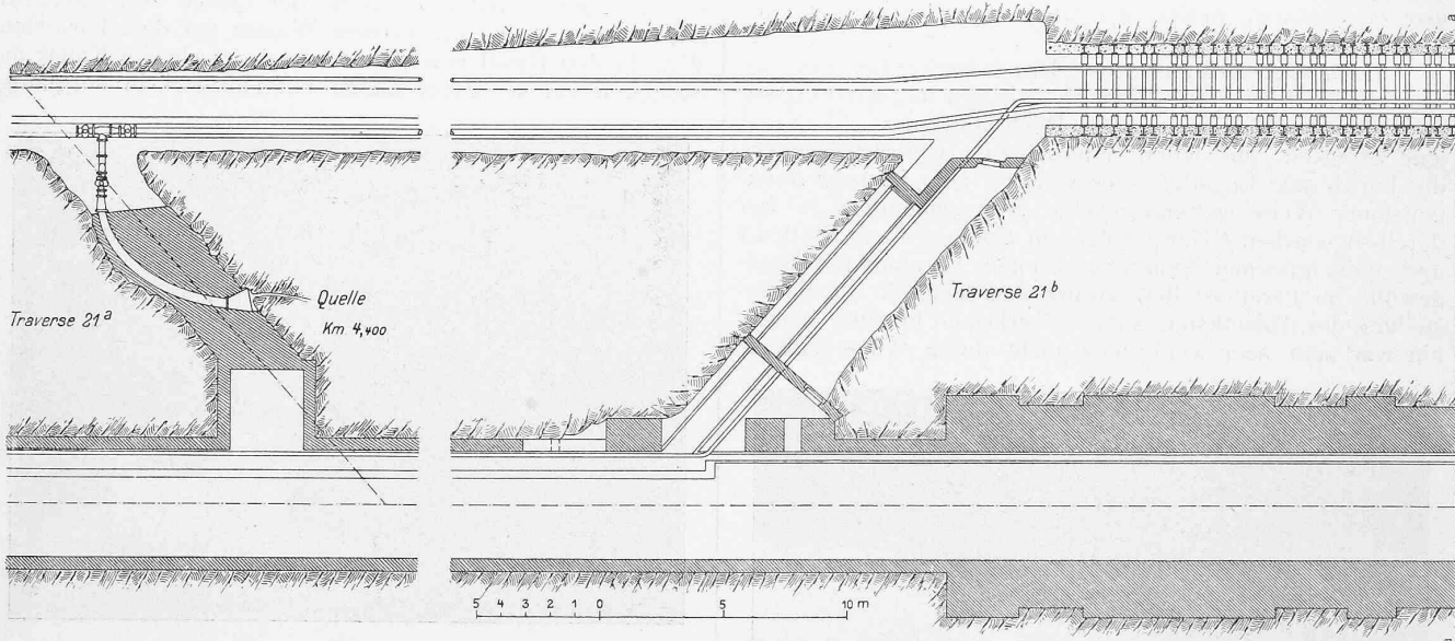
Abb. 56. Kuhlanlage. — Wasserfassung in Trav. 21 a. Presswasserbeschaffung durch Trav. 21 b mit Pumpenanlage in Trav. 23. — 1 : 300.
