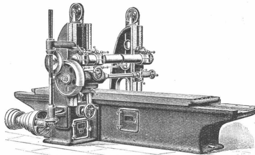
Plan-Fräsmaschine. No. 2.
