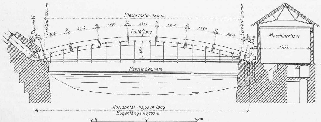
Abb. 10. Der selbsttragende Bogen am untern Ende der Druckleitung. — Masstab 1 : 400.
