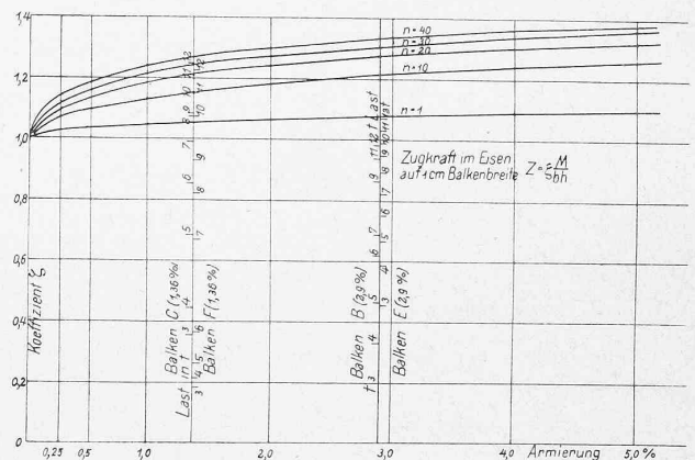
Abb. 6. Zugkraft im Eisen. Beton elastisch.
