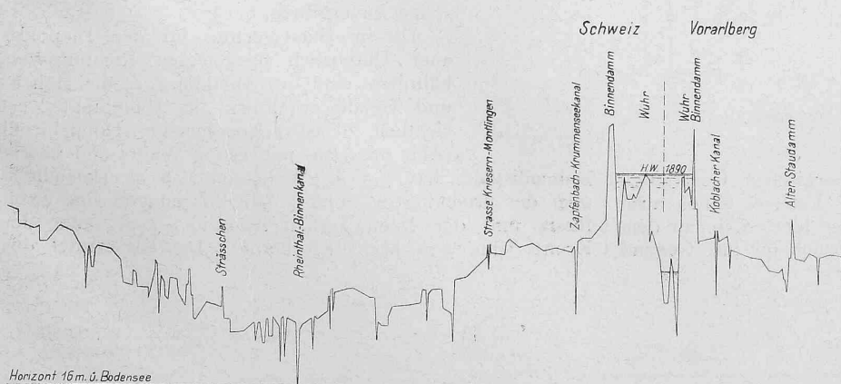
Abb. 6. Talquerprofil unterhalb Montlingen. — Masstab 1:25'000 f. d. L., 1:250 f. d. H.
