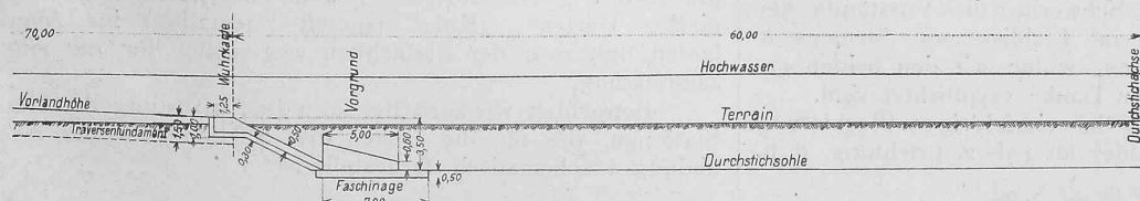
Abb. 8 b. Normalprofil laut Staatsvertrag, vom Wuhr bis zur Achse des Durchstiches. Masstab 1 : 500.
