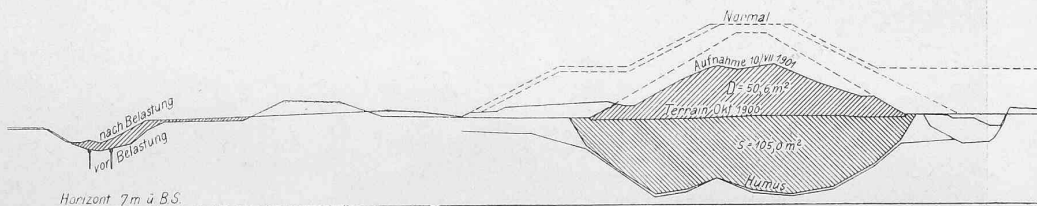
Abb. 10. Sondierungen am Versuchsdamme im Juli 1901 bei Hm 34 + 50. Masstab 1 : 500.
