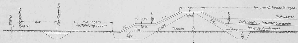
Abb. 8 a. Normalprofil laut Staatsvertrag.
