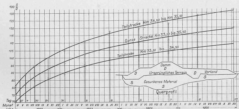
Abb. 31. Senkung des Probedammes.
