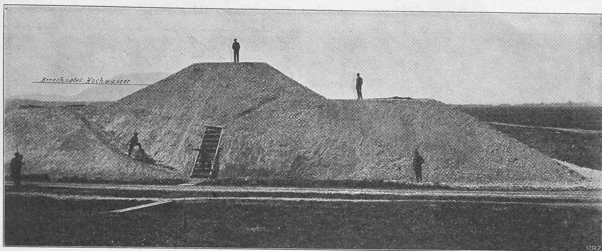
Abb. 30. Kopf des Probedammes beim Schwellengraben (von unten nach oben gesehen).
