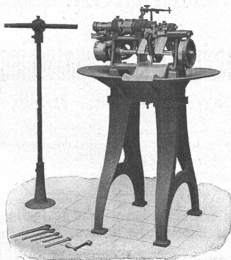
Automatische Façonbank.
