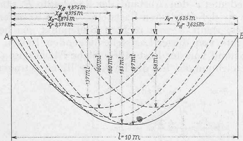
Abb. 4. Maximalmomentenkurve.
