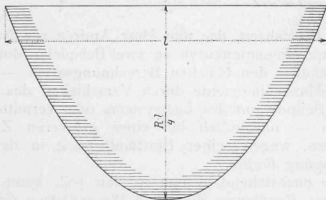
Abb. 5. Parabelschablone.
